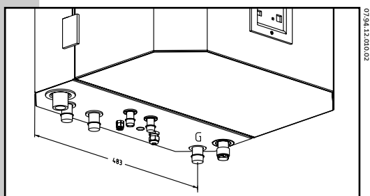
Figuur 16: Gasleidingaansluiting
