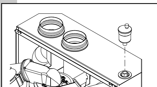
Figuur 14: Montage automatische ontlufter
