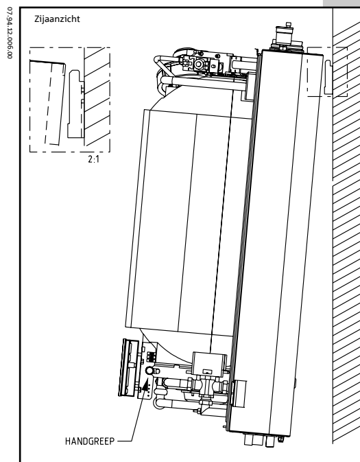
Figuur 10: Ophangingsindicaties
