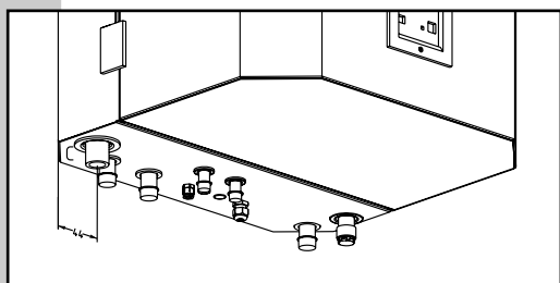
Figuur 21: Condensaansluiting
