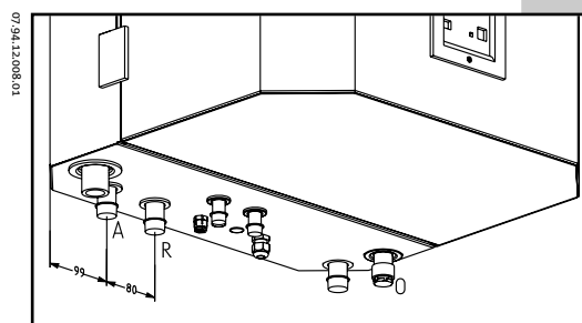
Figuur 11: Cv-aanvoer- en retourleidingen
