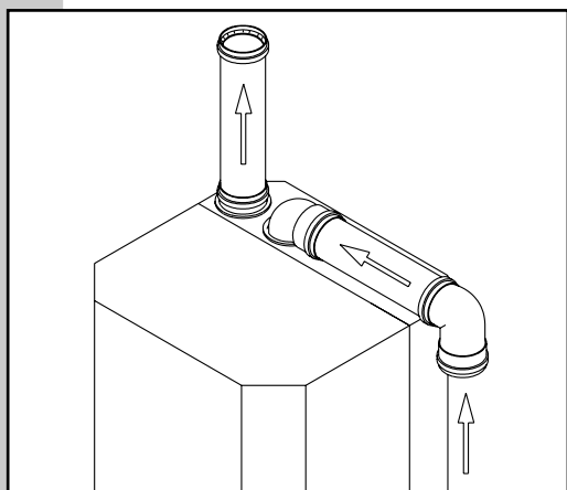
Figuur 24: Luchtinlaatzijde
