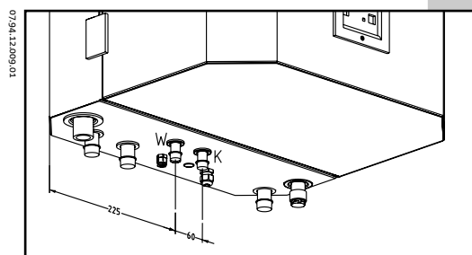
Figuur 15: Sanitairzijdige warm- en koudwateraansluiting
