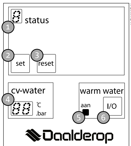
Figuur 4: Bedieningspaneel
